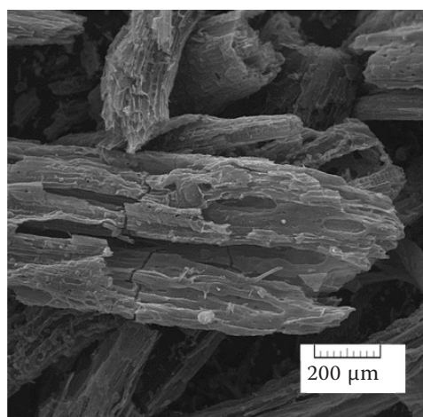
SEM HV: 30.00 kV WD: 10.18 mm View field: 1.24 mm Det: SE SEM MAG: 175 × Date (m/d/y): 09/11/15
